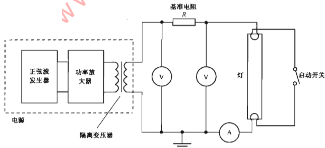
图5 高频基准线路
